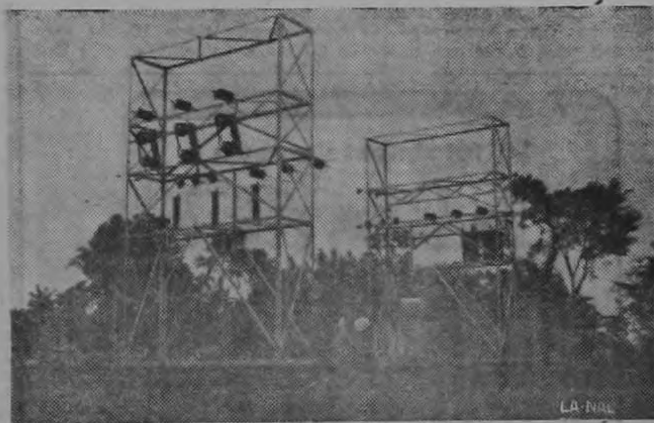
Sub Estación de Esparta. Recibe corriente de Nagatac, y la transforma para uso de la población. Costo: ₡ 19.000.00
