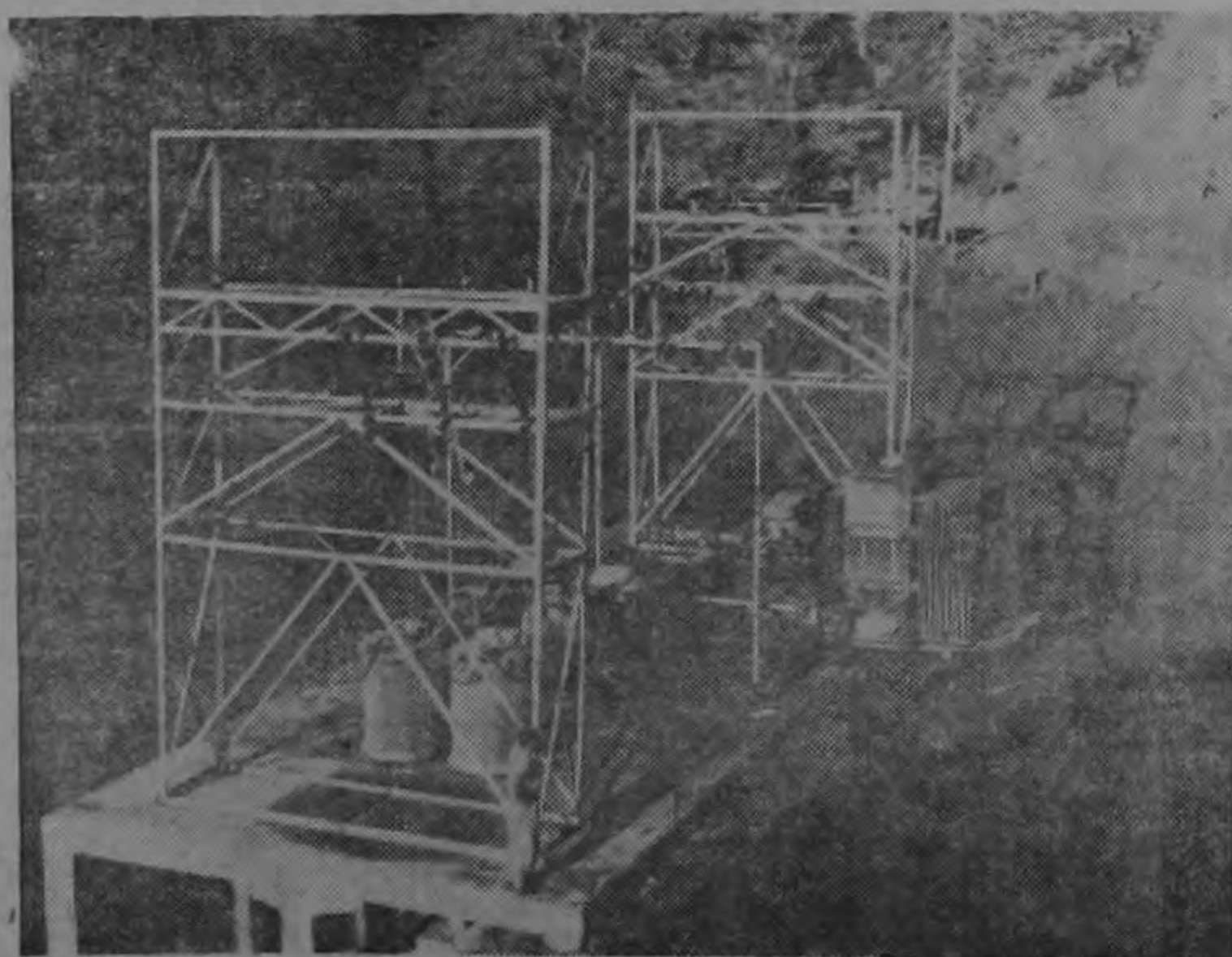
Sub-Estación de Nagatac. Eleva a 33 mil voltios la corriente producida por la Planta del mismo nombre, y la transmite a Esparta, Barranca, y Puntarenas. Costo: ₡75.000.00.
