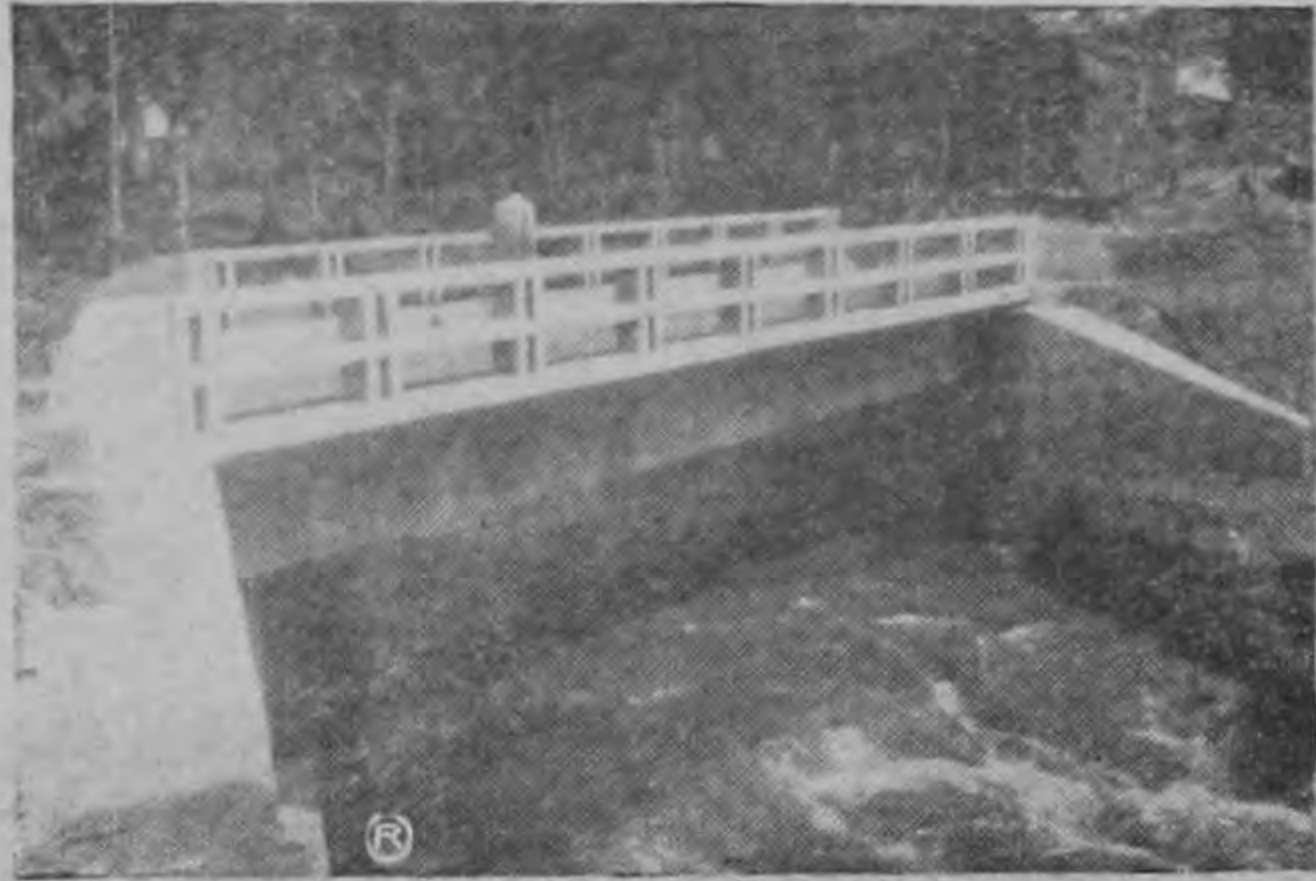
MODERNO PUENTE CIEGO EN QUEBRADA AZUL CONSTRUYE EL M.O.P.—El Ministerio de Obras Públicas, continúa su empeñosa labor de construcción de puentes para mejorar la comunicación y dar salida a los productos agrícolas, de las regiones productoras como en el Cantón de San Carlos. En Quebrada Azul se ha terminado la construcción de un puente ciego, que se aprecia en esta foto. El puente ciego consiste en una construcción en tierra firme al lado del cauce natural, después de haberlo desviado.
