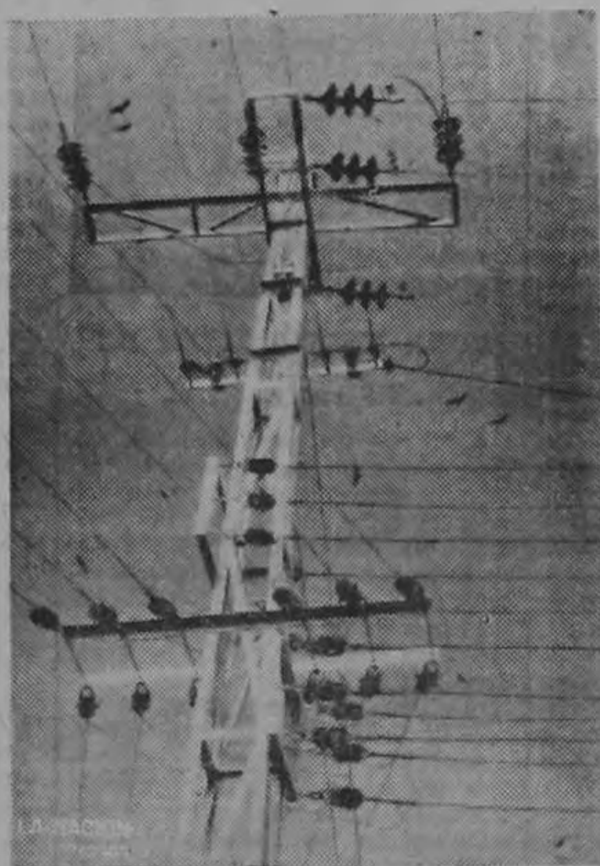
de entrada a la Sub-Estación de Puntarenas. Líneas de 33.000 voltios y de 2400 se ven en la gráfica
